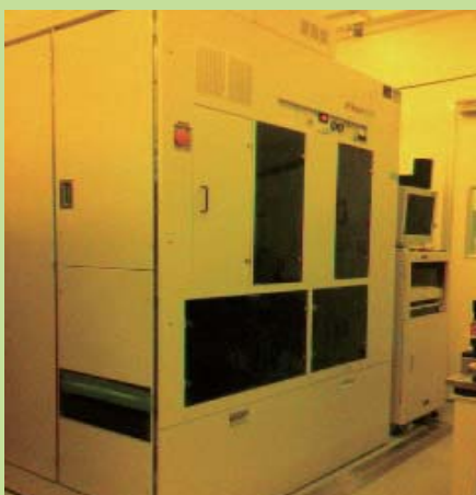
i線 - ステッパー 8インチ
