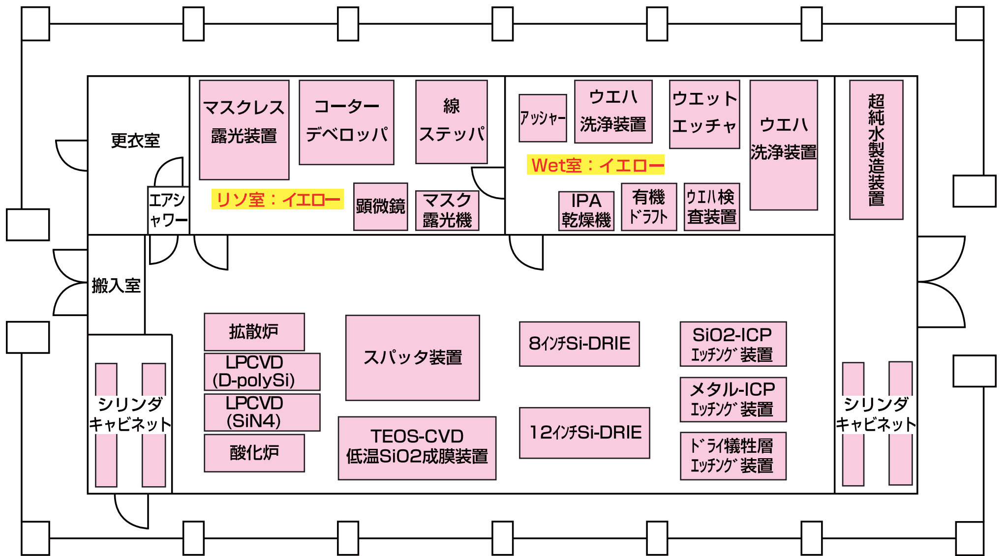
TKB812F設備配置図(約350m 2 、クラス1000)
